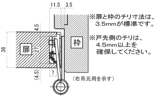
下用(右)丁番
