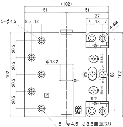
下用(右)丁番
