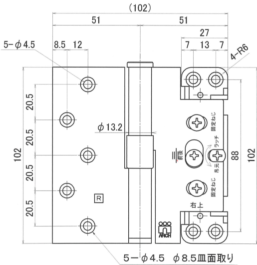
上用(右)丁番
