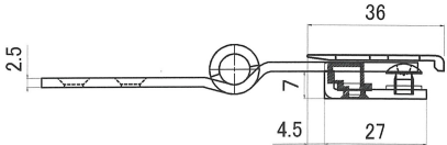
上用(右)丁番
