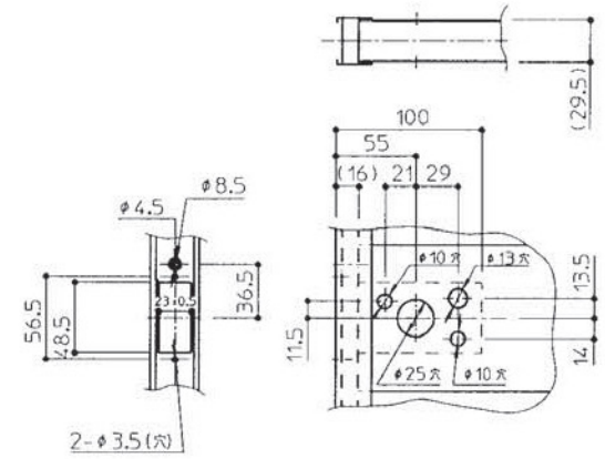
取付穴寸法
