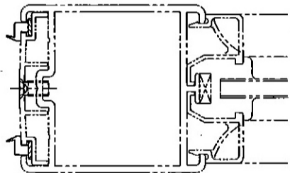
片開き納まり図 (Scale 1/1)
