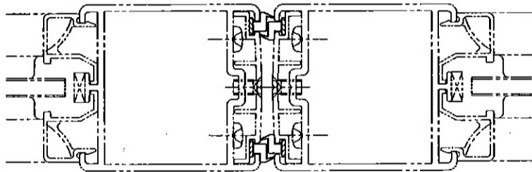
△ 引分け納まり図 (Scale 1/1)
