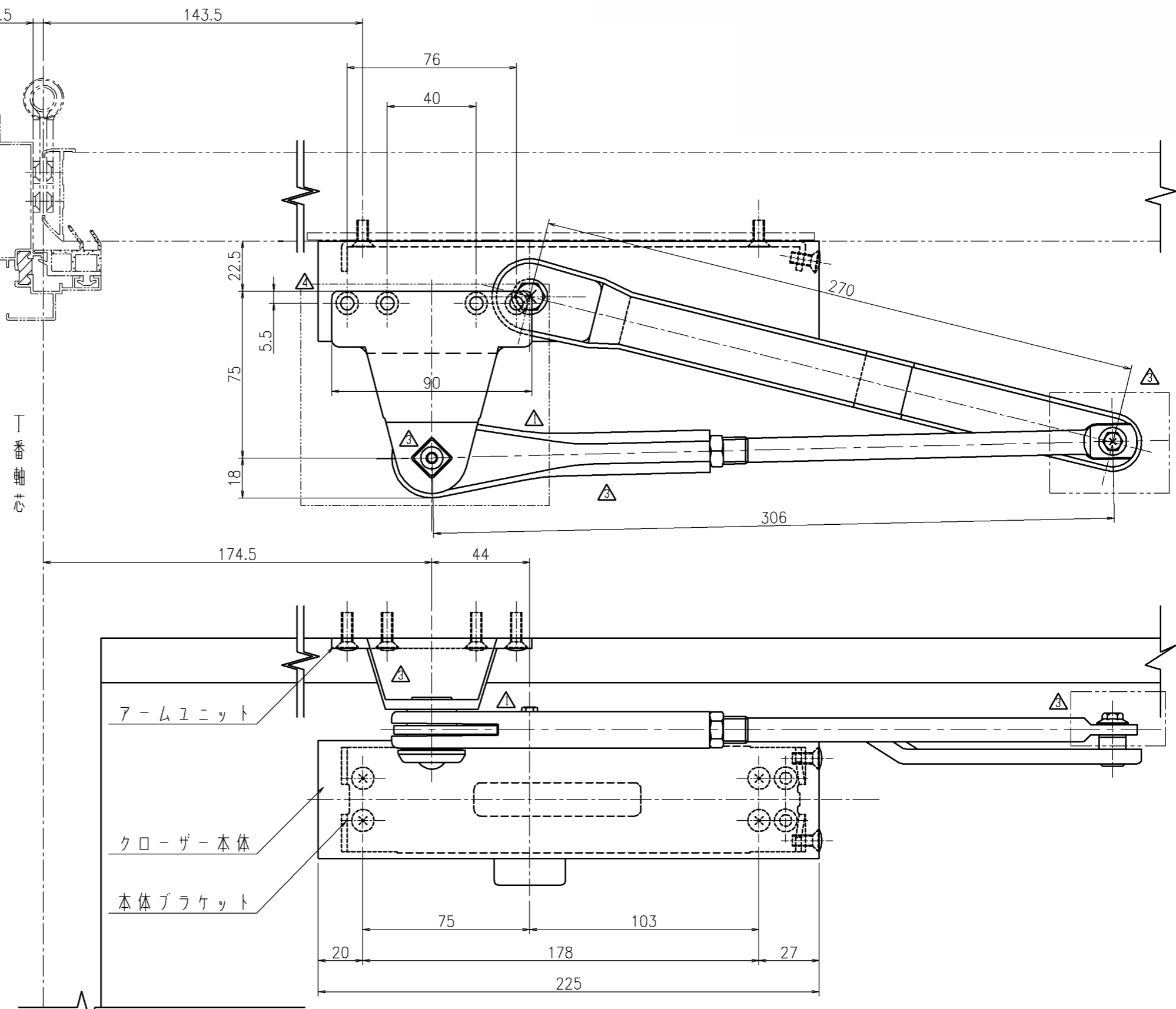
E X II 納まり図
