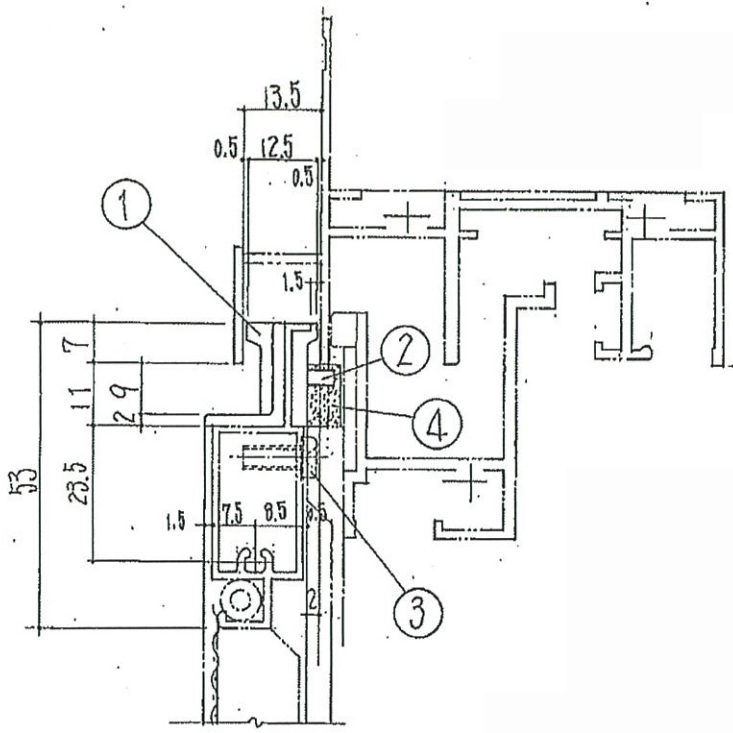
取付位置 (内観図)
