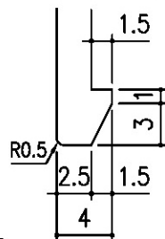
D部詳細図 S=2/1
