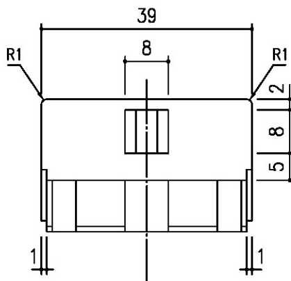
D部詳細図 S=2/1
