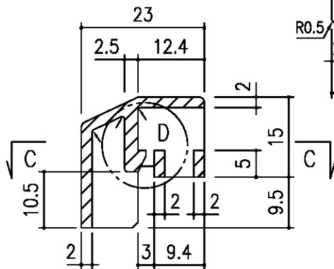
B-B 断面图
