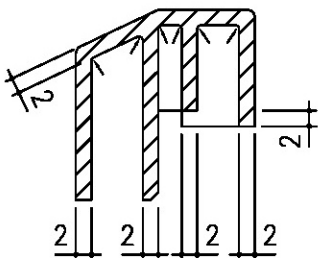
A-A 断面图
