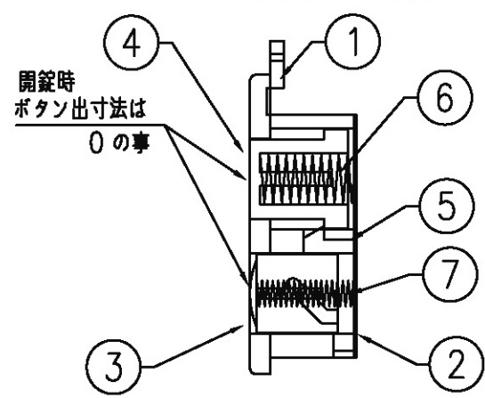
A-A断面図 (開錠時)
