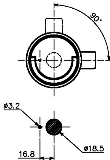
左吊りパネル切欠図
