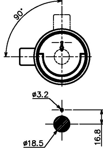
右吊りパネル切欠図
