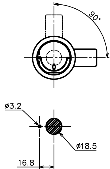
左吊りパネル切欠図
