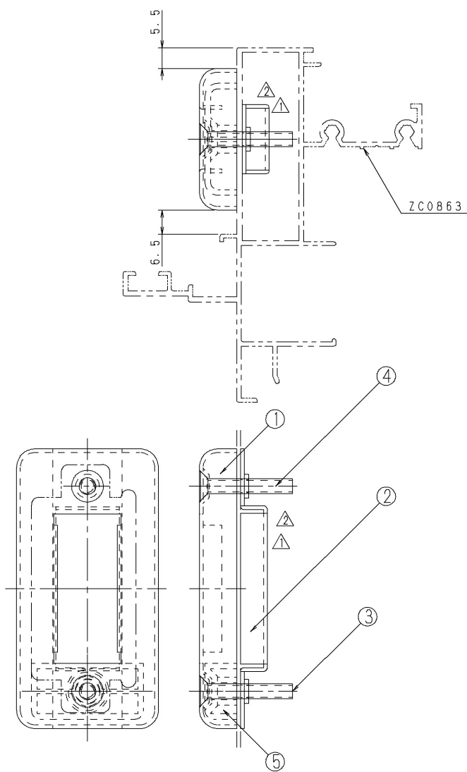
縦枠の納まり図 (1:1)
