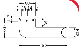
H=24mm 本図は左勝手
