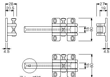
ストップ付 No.1540-CS
