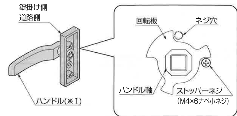
ストッパーネジの取付パターン表 ※図は両錠タイプですが、片錠タイプも同様です。
