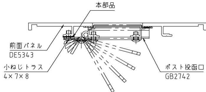
納まり図 (1:2)
