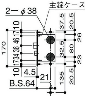
扉切欠図
