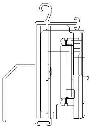
(取付状態図)
