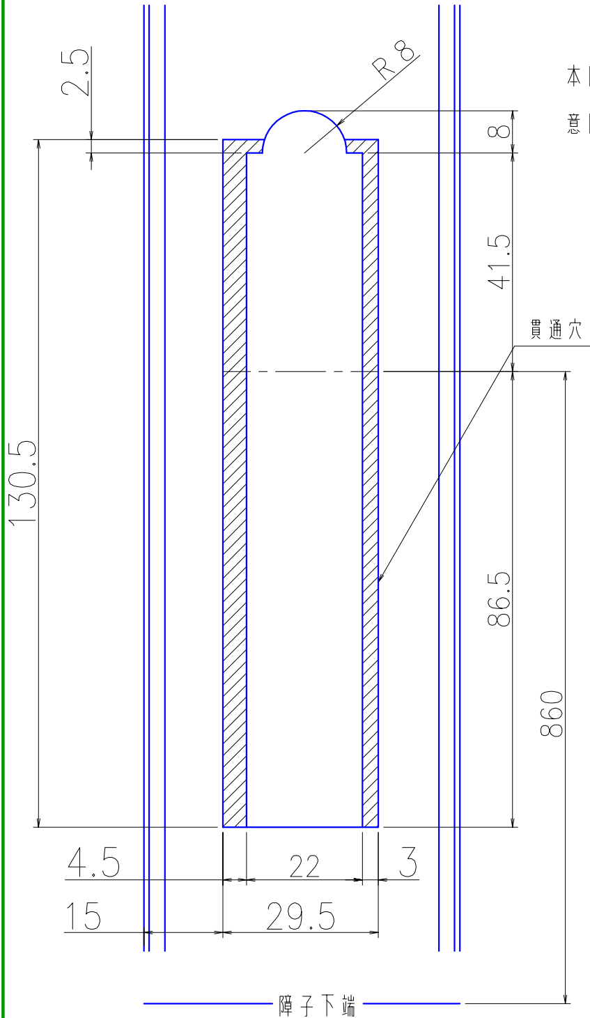
戸当り框又は突合せ框（右）の貫通穴
