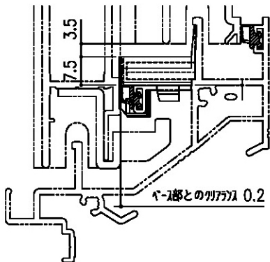
納まり図 (S=1/1)
