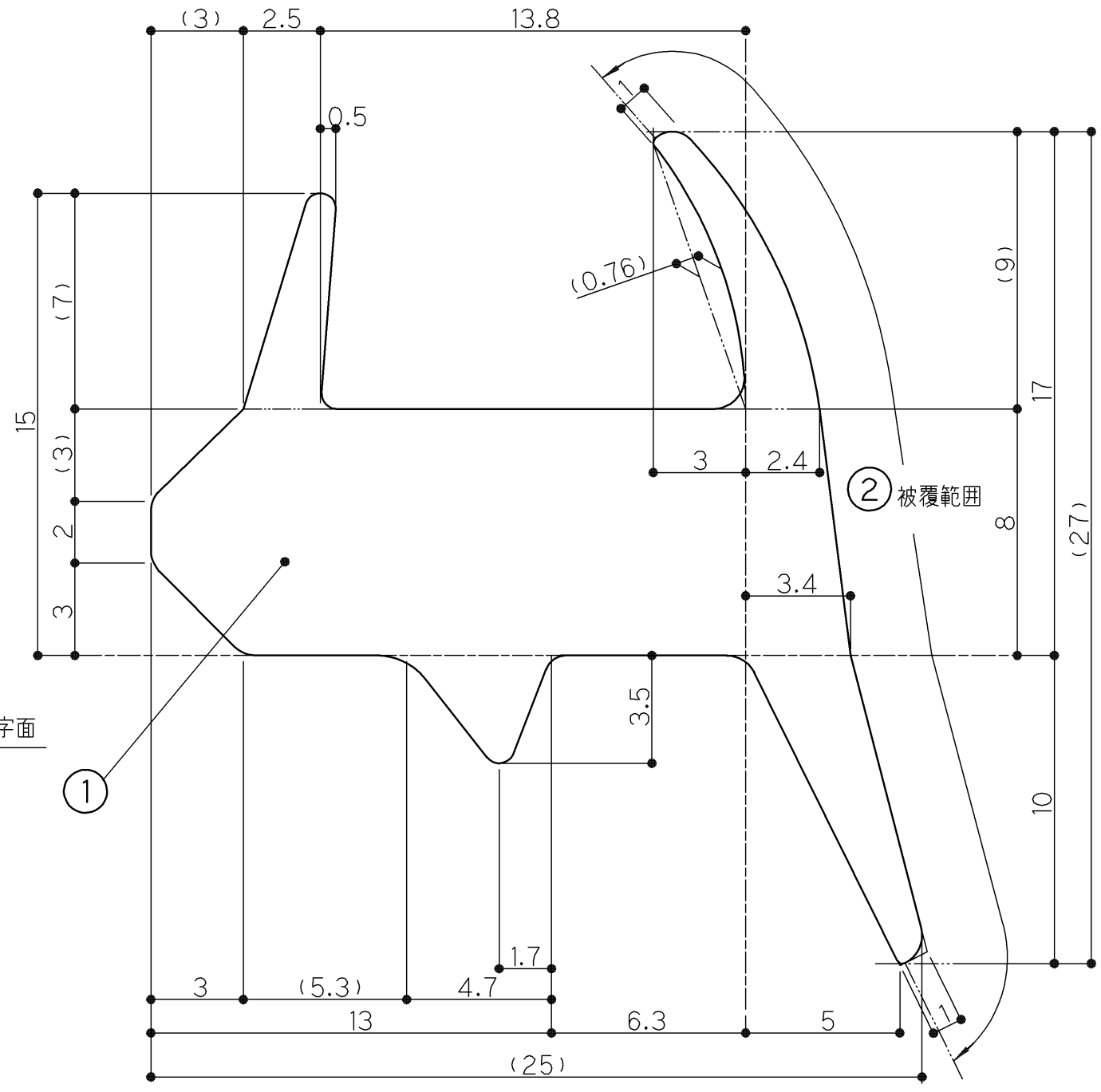
断面 (S=5/1)
