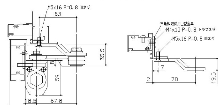
③ 参考納まり図（エルコン3型の場合）
