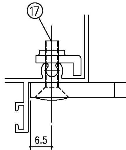
A 部 詳細図
