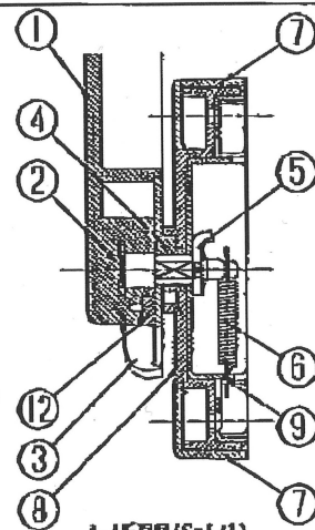
A-A断面図 (S=1/1)
