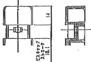
ピストンキャップ図放図 (S=1/1)
