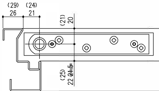
取付け図 (1/2)
