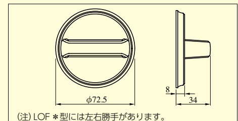
戸襖錠の外形寸法図
