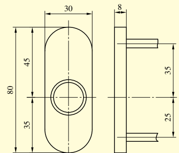
バックセット31mm用ハンドル座
