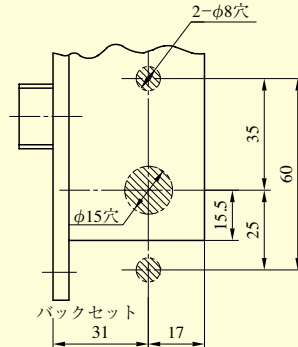
バックセット31mmの レバーハンドル部の切欠
