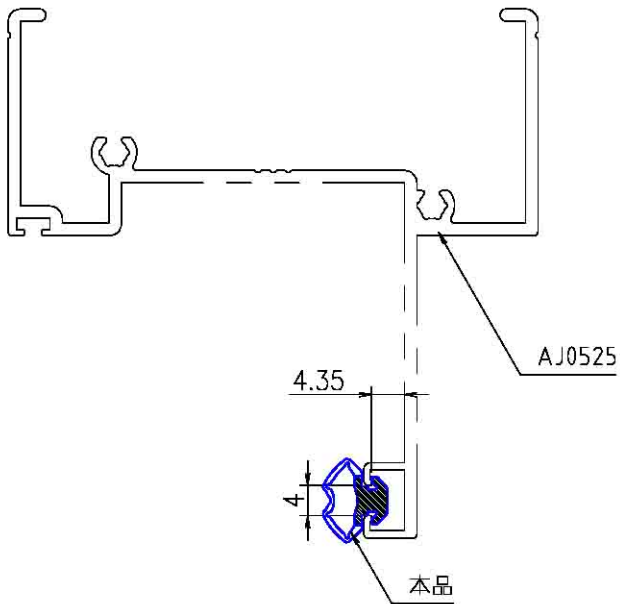
納まり図 (1:1)
