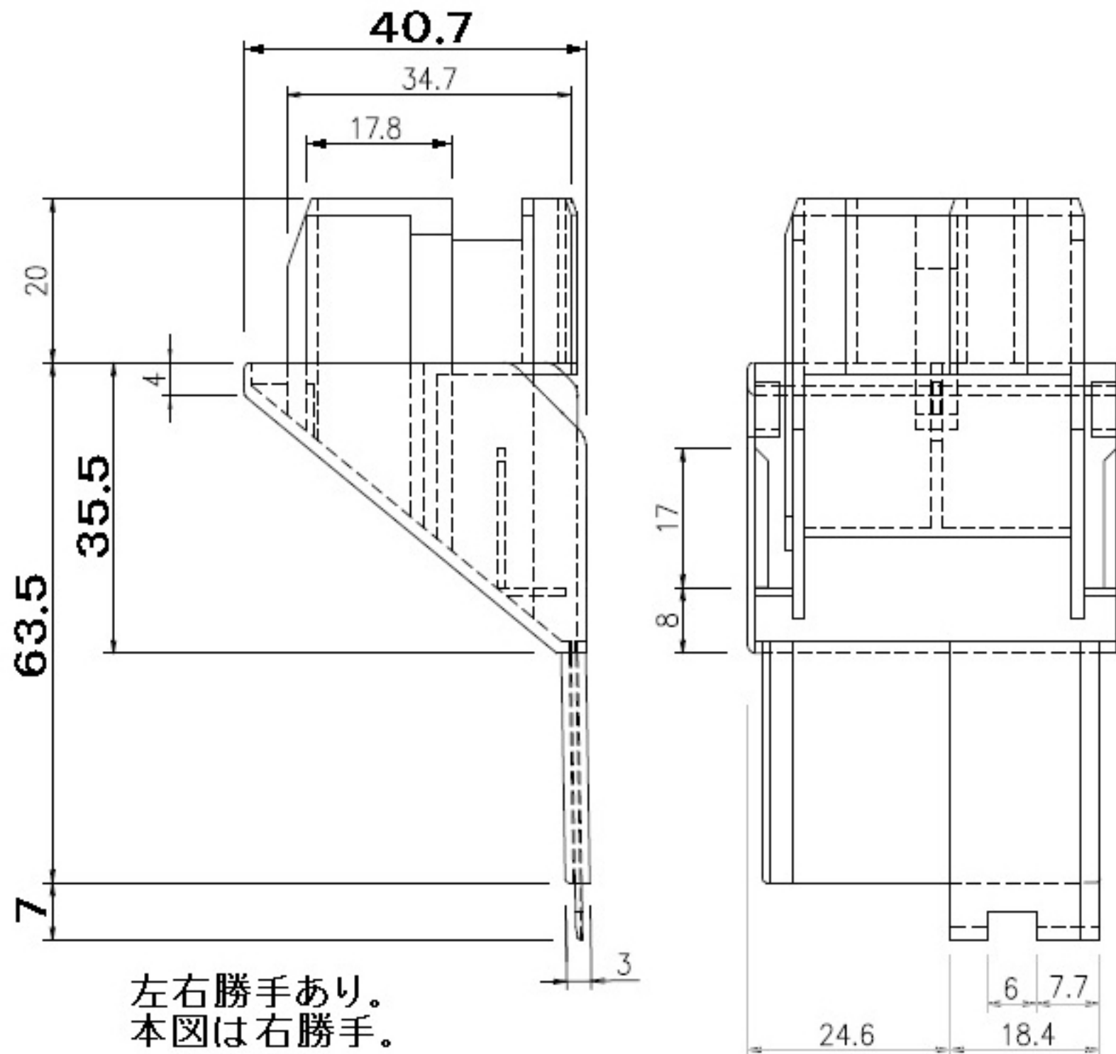
MTG-70 (14) 引違い窓 小口キャップ(下) BBJ243
