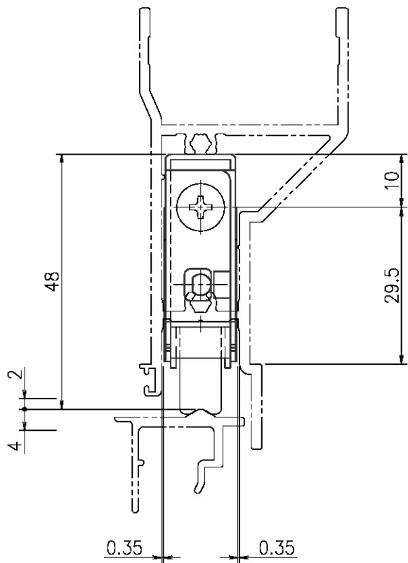
納まり図 (1:1)
