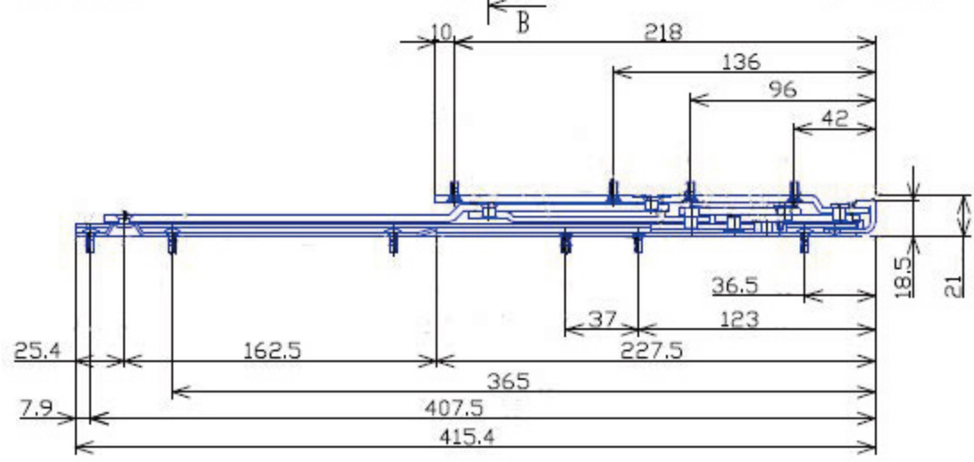
A-A断面
