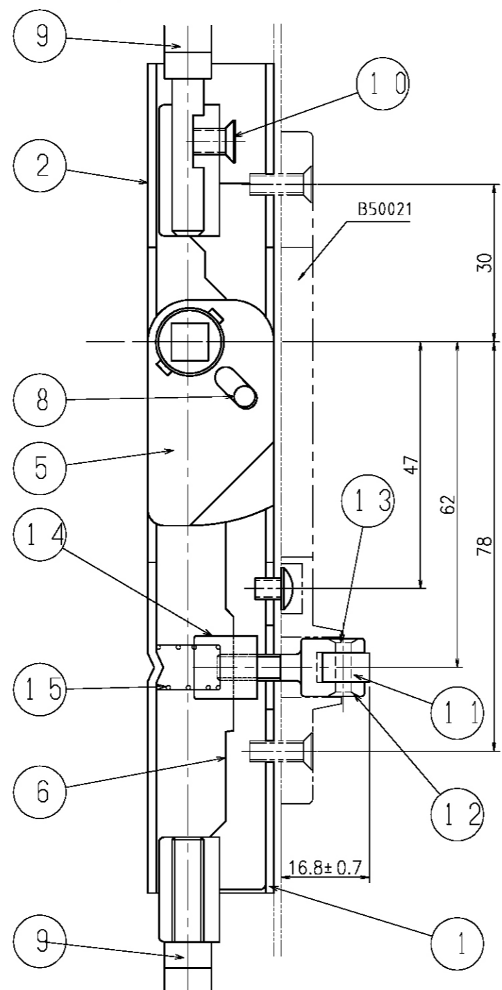
A 矢視図
