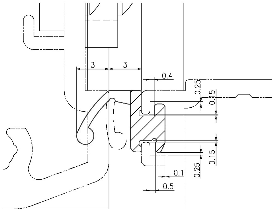
△ 納まり図 (5:1)
