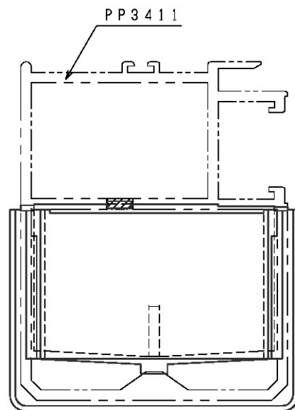
納まり図 (1:1)
