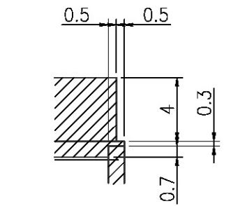
A 矢视图 (3:1)
