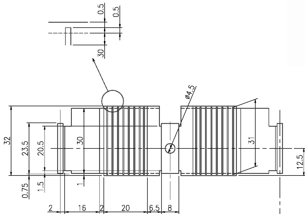
A 矢视图 (3:1)
