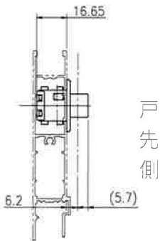
△ 納まり図 (1:2)
