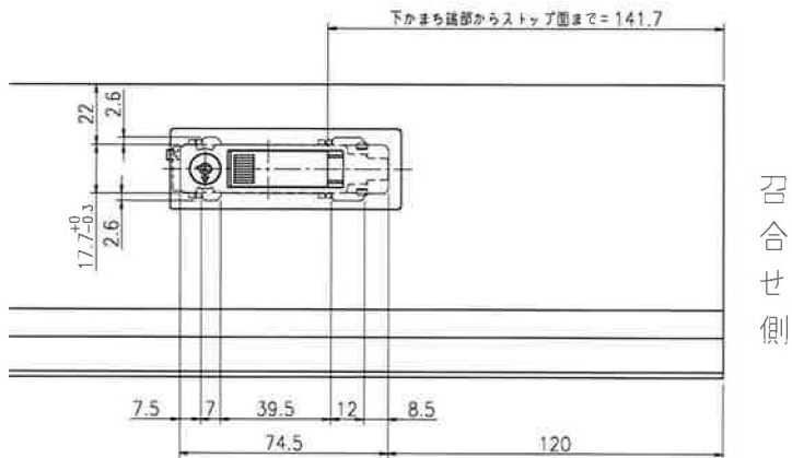
△ 納まり図 (1:2)
