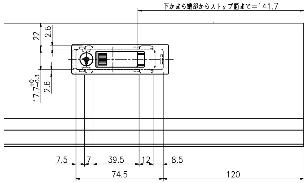
納まり図 (1:2)
