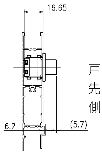
納まり図 (1:2)
