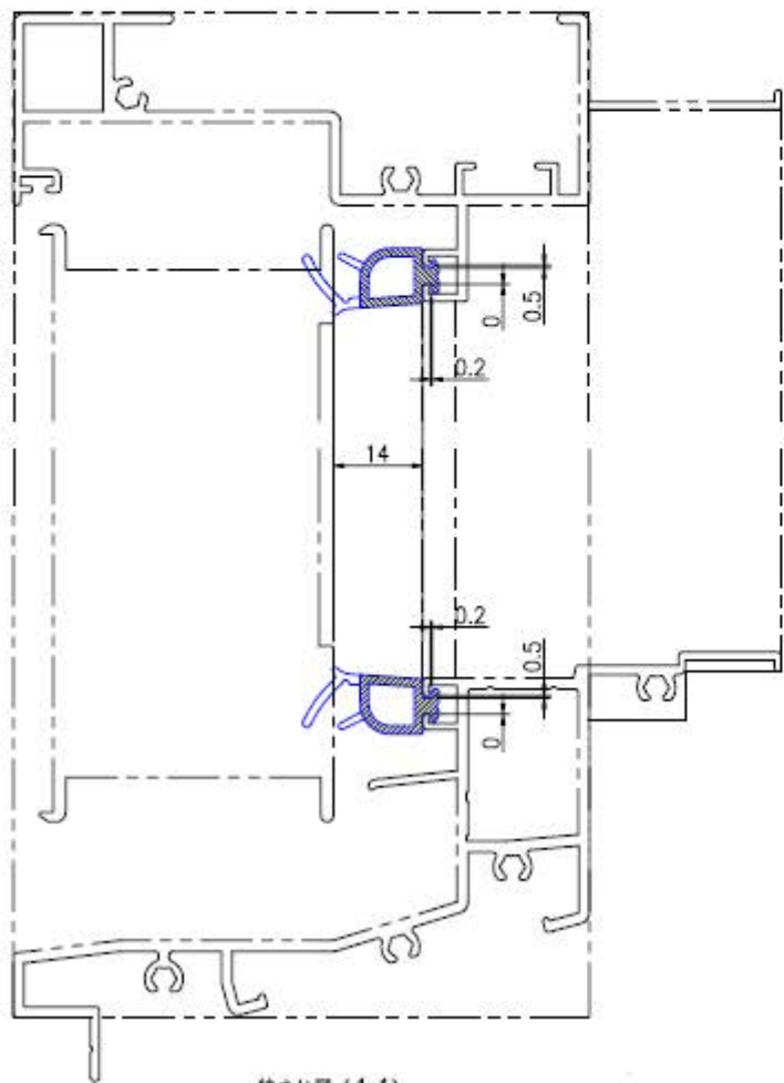
納まり図 (1:1)
