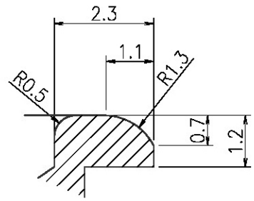
B部詳細 (4:1)
