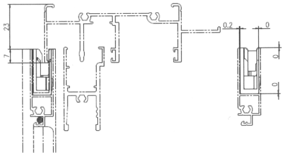
納まり図 (1:1)
