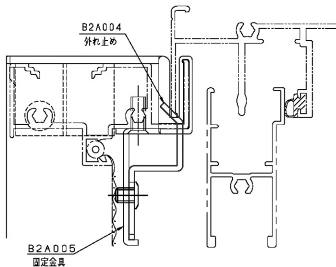
取付状態図(1:1)
