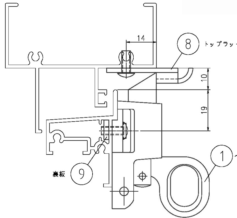
納まり図 (1:1)
