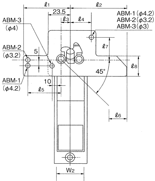
■ 取付け穴寸法 Dimension of mounting hole
