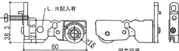
偏芯戸車
