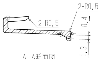
A-A断面图
