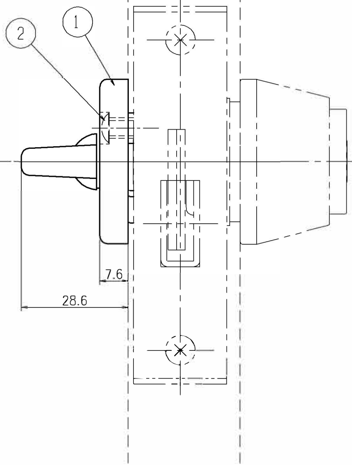
サムターン 納まり図 (1:1)
