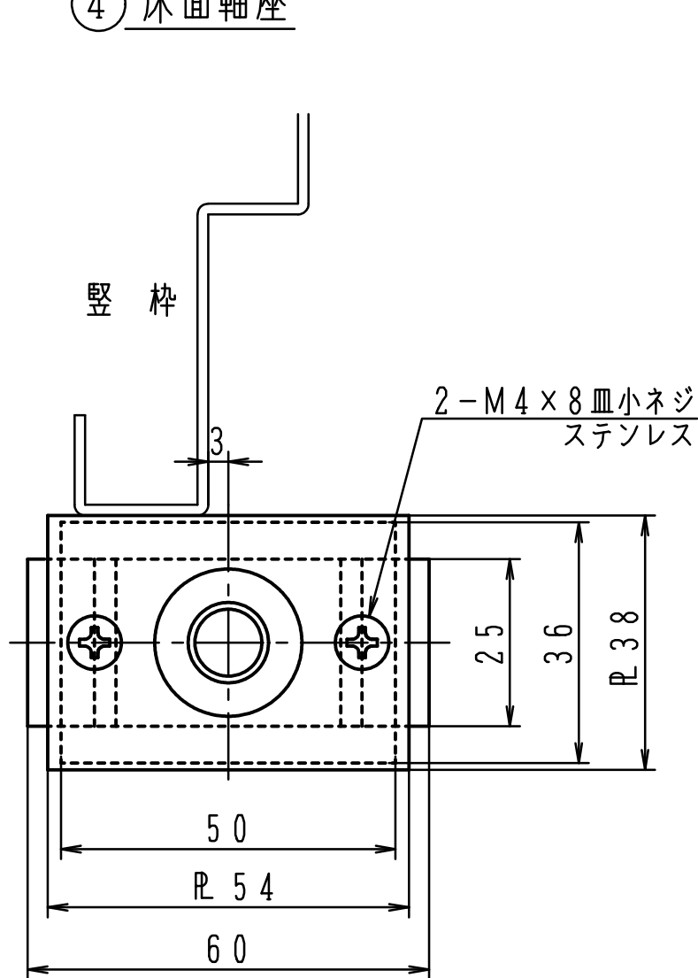
④ 床面軸座
