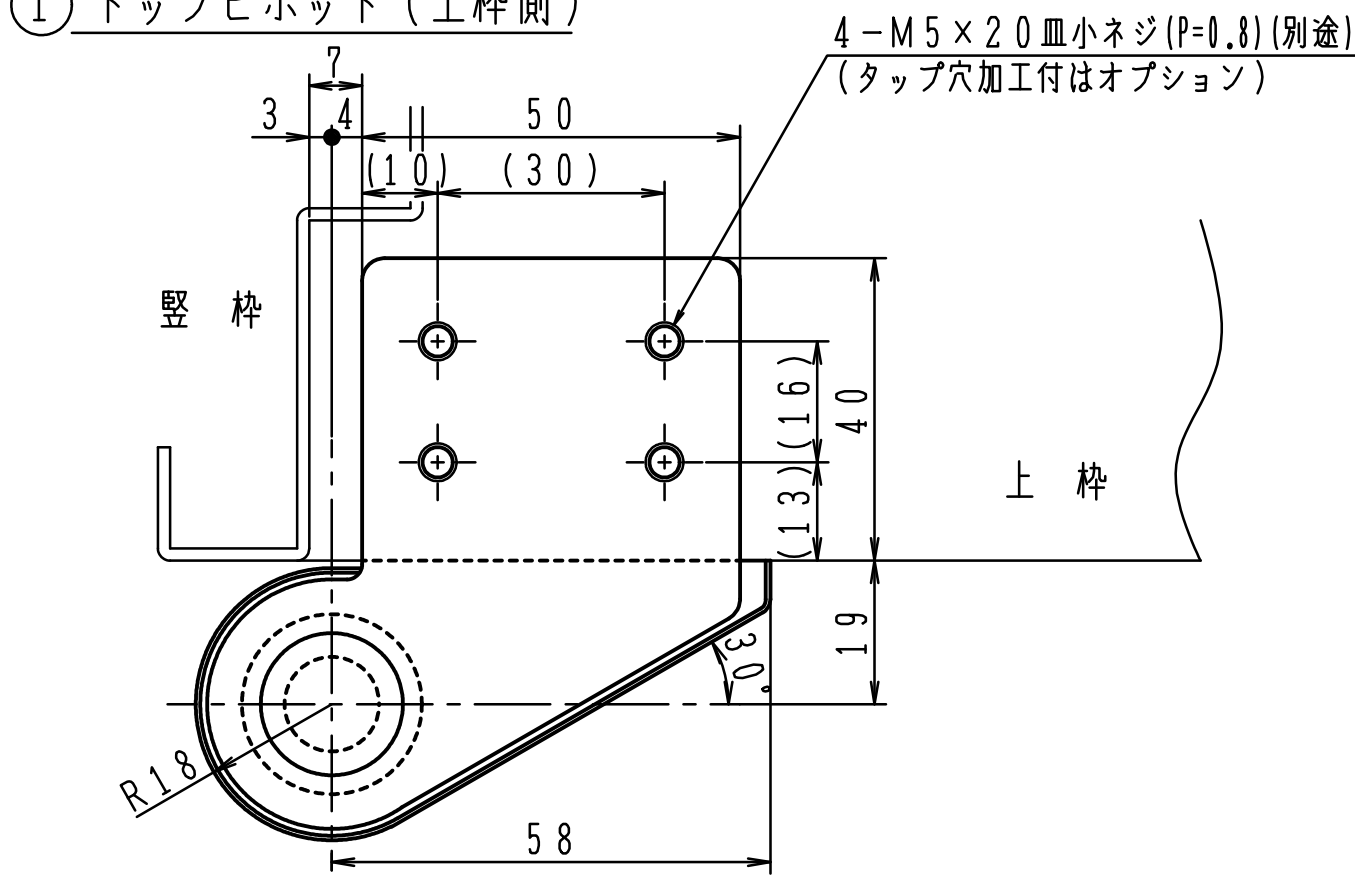
① トップピボット（上枠側）
