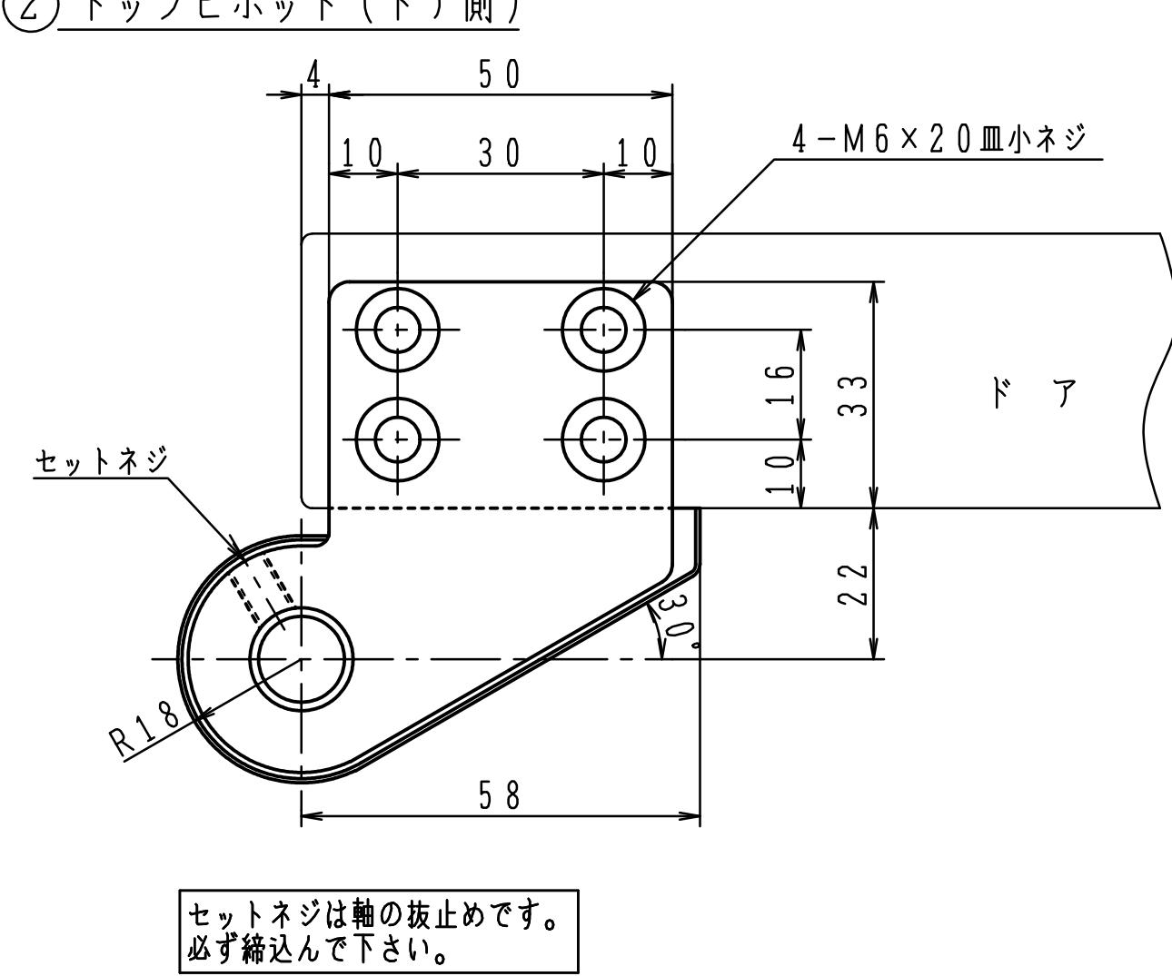
② トップピボット（ドア側）
